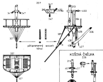
KOŠ HLAVNĚHO STĚŽNĚ
