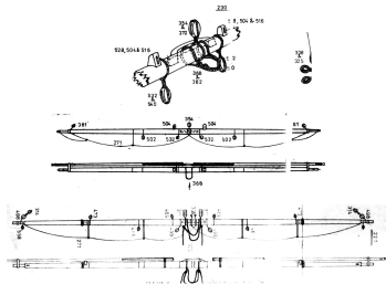
RAHNA HLAVNĚHO STĚŽNĚ
