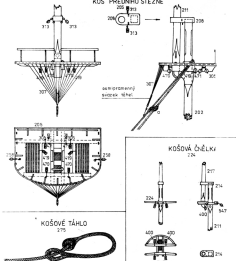
KOŠ PŘEDNĚHO STĚŽNĚ
